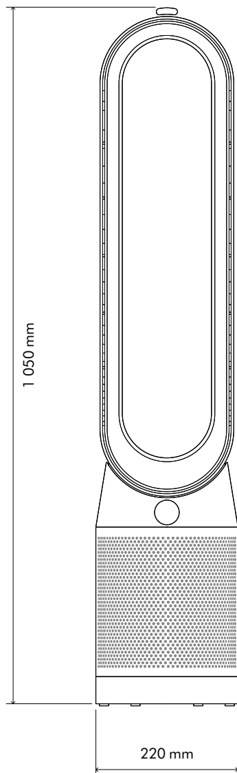
Plan d'élevation
