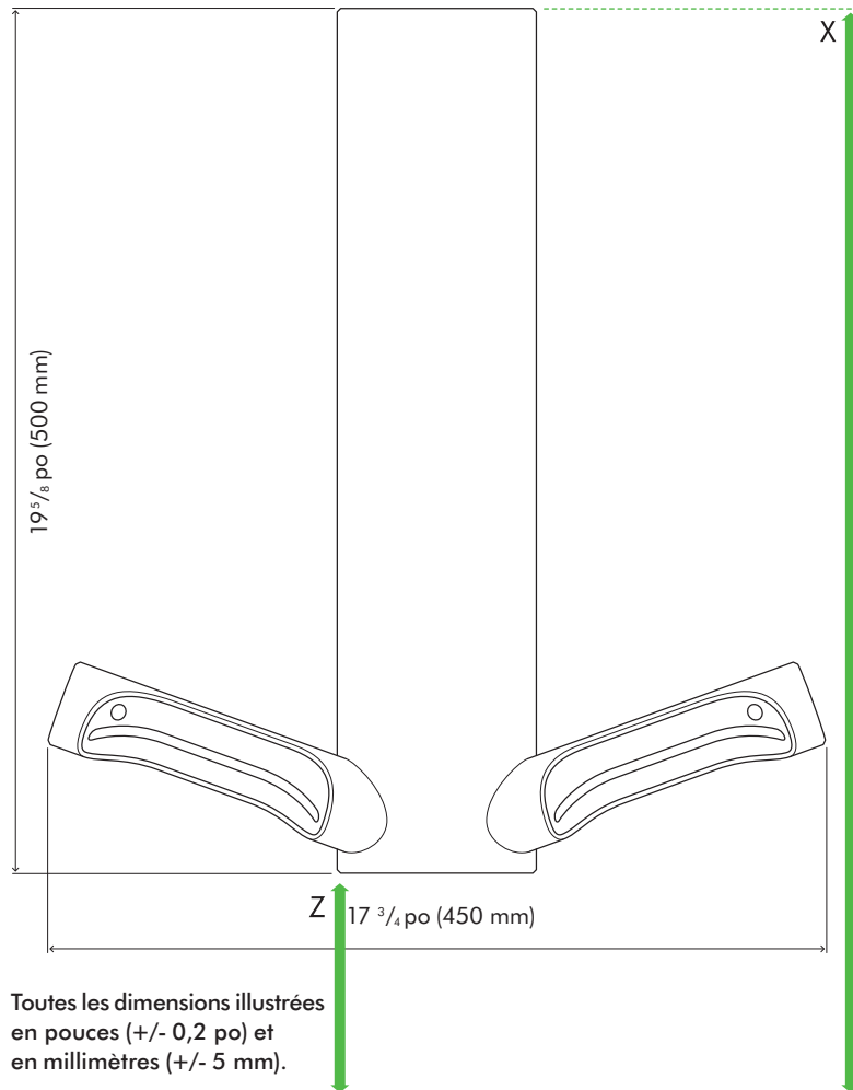
Élévation avant
