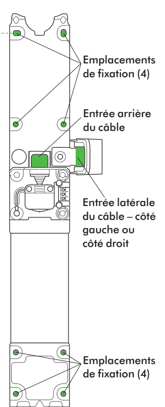
Plaque arrière
