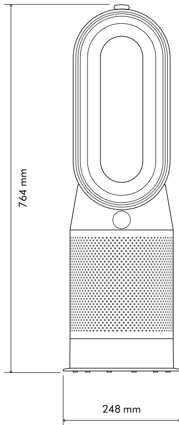
Plan d'élevation
